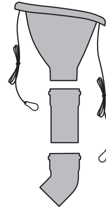
Conjunto de embudo y tubería de entrada
